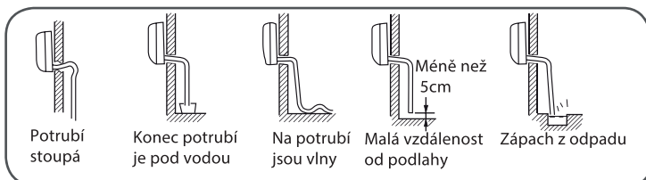
Vnitřní jednotka
